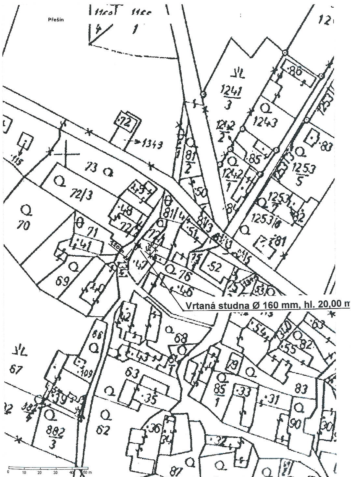
Příloha 2.3 Situace umístění studny M 1 : 1000
