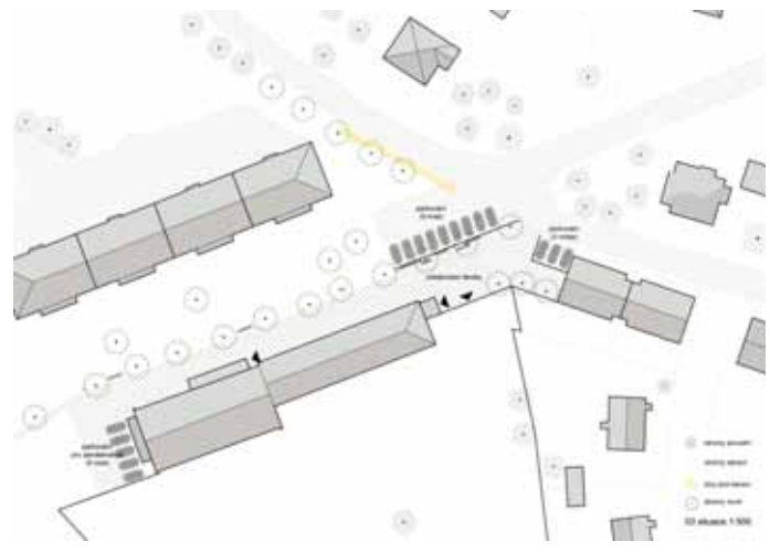
Půdorys a vizualizace návrhu severního předpolí MŠ Nepomuk (City Upgrade).
