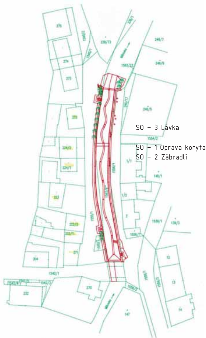
Půdorys nové úpravy dle projektové dokumentace
